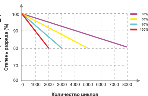
Зависимость циклов от глубины разряда
